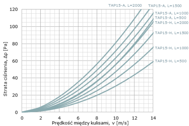
Wykres 2. Straty ciśnienia tłumika TAP-15.
