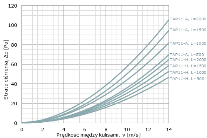
Wykres 1. Straty ciśnienia tłumika TAP-11.
