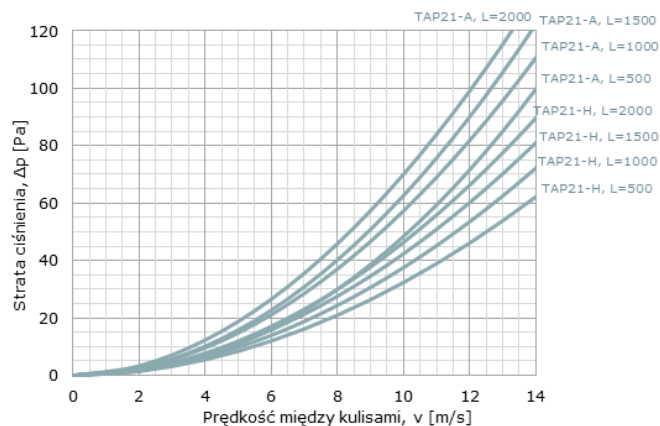
Wykres 4. Straty ciśnienia tłumika TAP-21.
