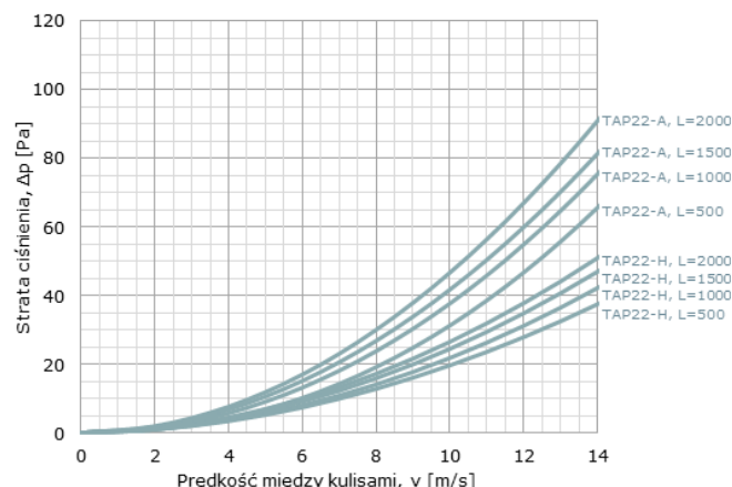
Wykres 5. Straty ciśnienia tłumika TAP-22.
