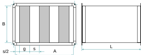
Rysunek 1. Wymiary tłumika TAP
