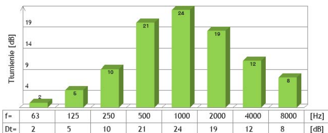
Rysunek 6. Przykład doboru tłumika TAP
