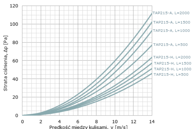
Wykres 3. Straty ciśnienia tłumika TAP-215.
