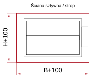
Rysunek 2. Wymagane otwory dla kłapy KWP-P montowanej pojedynczo.
