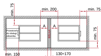
Rysunek 4. Wymagane odległości między kłapami montowanymi pojedynczo.
