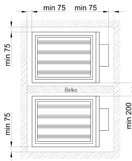
Rysunek 3. Wymagane odległości między kłapami.
