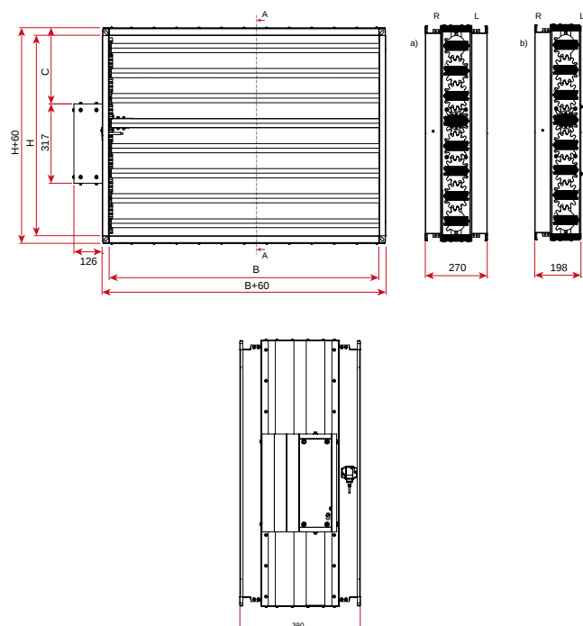
Rysunek 1. Wymiary kłap WKZ-O (z ramkami przyłączeniowymi po obu stronach).
